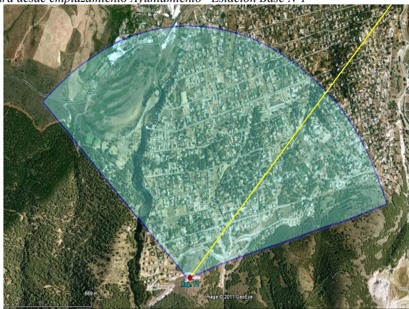
Cobertura desde emplazamiento Repetidor de T.V. – Estación Base Nº2
