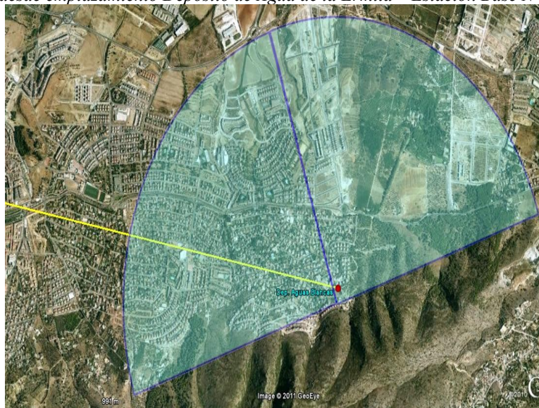
Cobertura de los sectores Wimax del emplazamiento Depósito de Casas Blancas – Estación Base Nº4
